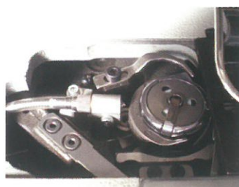
水平釜用 for vertical-axis hook
